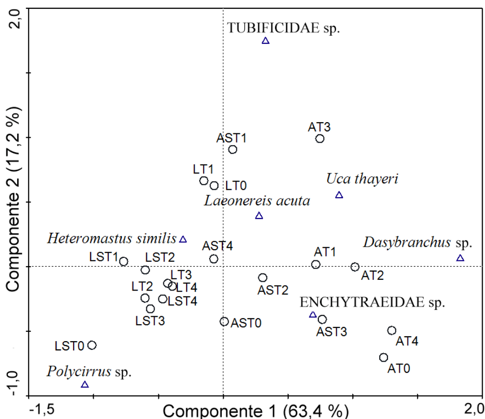
Figura 4 – Resultado da Análise de Correspondência com os agrupamentos dos táxons da macrofauna bentônica selecionados segundo o pressuposto de normalidade. Legenda: A: areia; L: lodo; T: toca; ST: sem toca; O: amostra central; 1: amostra adjacente 1; 2: amostra adjacente 2; 3: amostra adjacente 3; 4: amostra adjacente 4.
